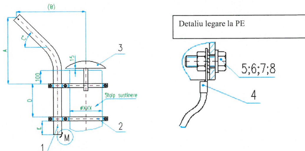
Fig.1-montarea consolei cu coliere pe stâlp: 1 - braț consola ; 2- sistem de prindere; 3- capac stâlp; 4- conductor
